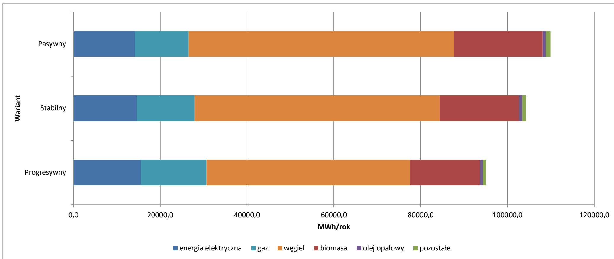
Rysunek 20. Perspektywiczne zużycie energii z podziałem na poszczególne rodzaje paliw i nośników energii dla roku 2034.
