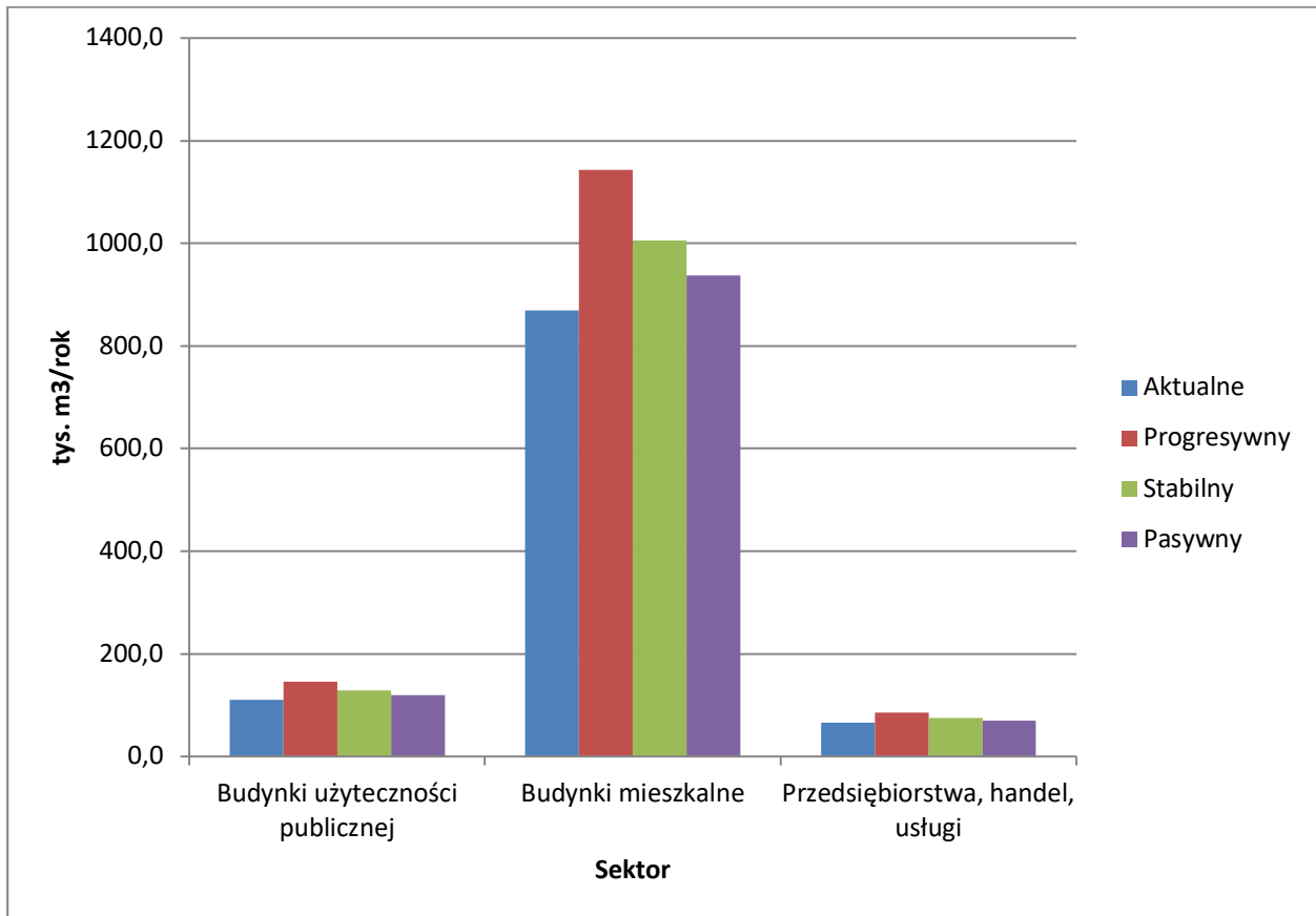
Rysunek 17. Szczegółowy bilans rocznego zapotrzebowania na paliwa gazowe na terenie Gminy Twardogóra.
