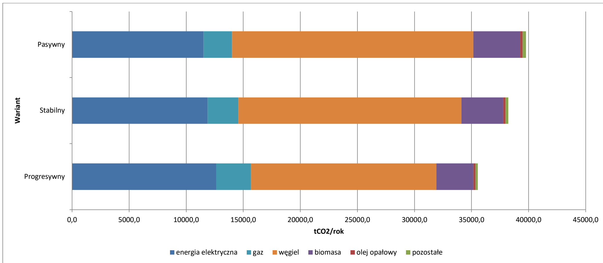
Rysunek 21. Perspektywiczna emisja CO 2 z podziałem na poszczególne rodzaje paliw i nośników energii dla roku 2034.
