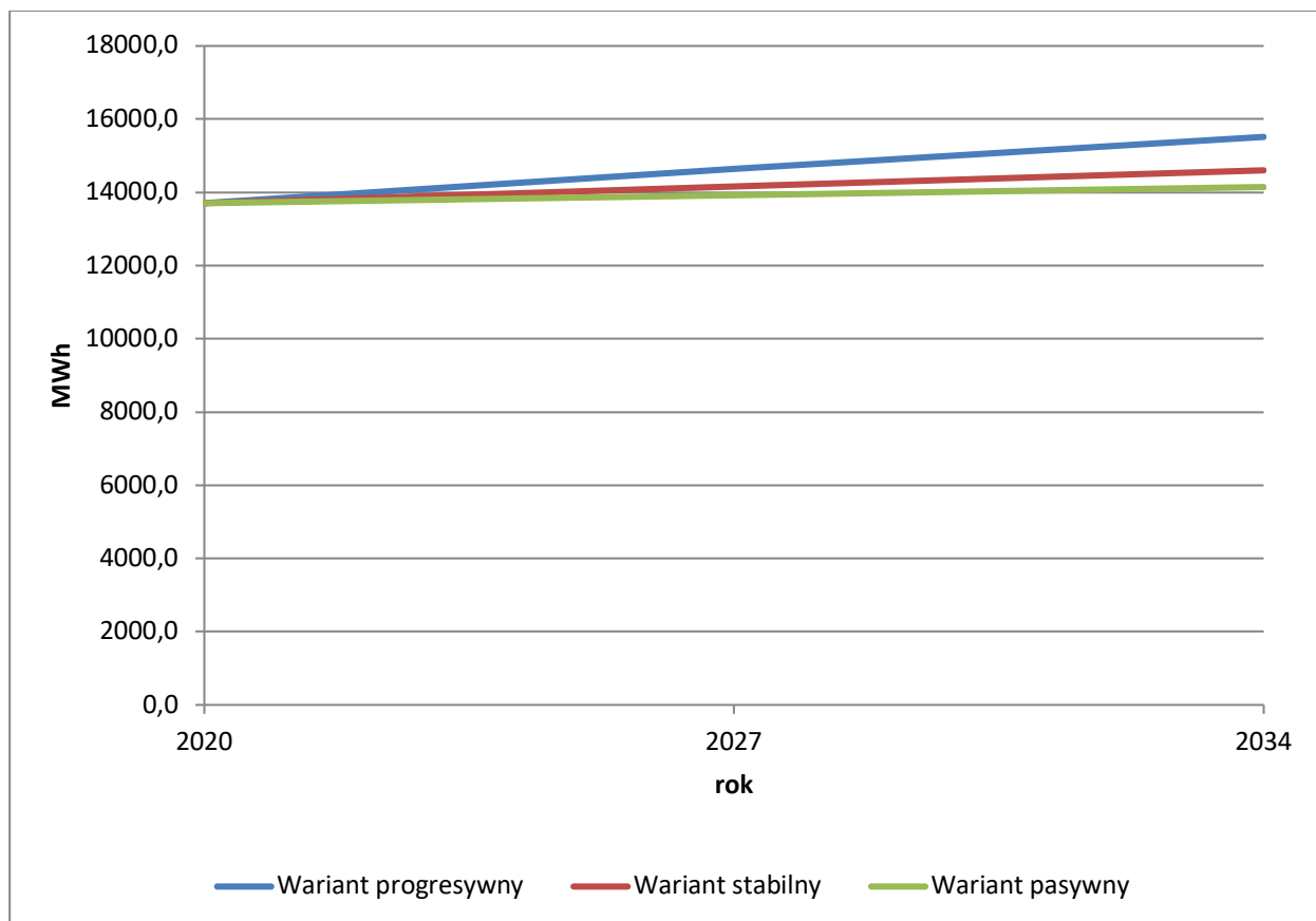
Rysunek 14. Prognozowana zmiana rocznego zużycia energii elektrycznej do roku 2034.
