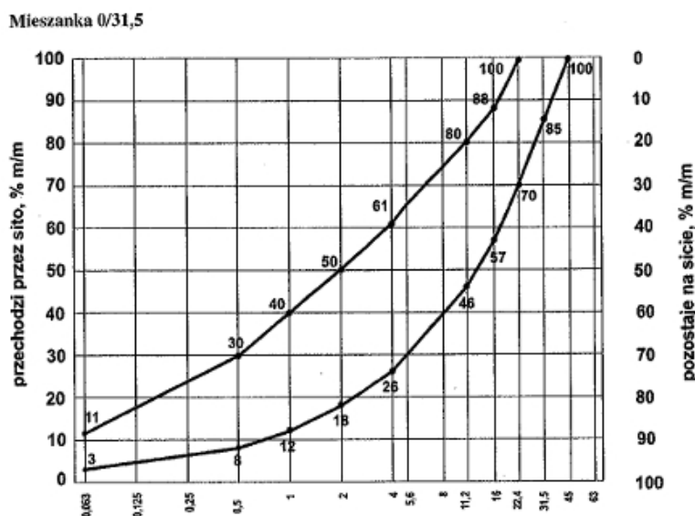
Rys. 2. Krzywe graniczne uziarnienia dla kruszywa 0/31,5.
