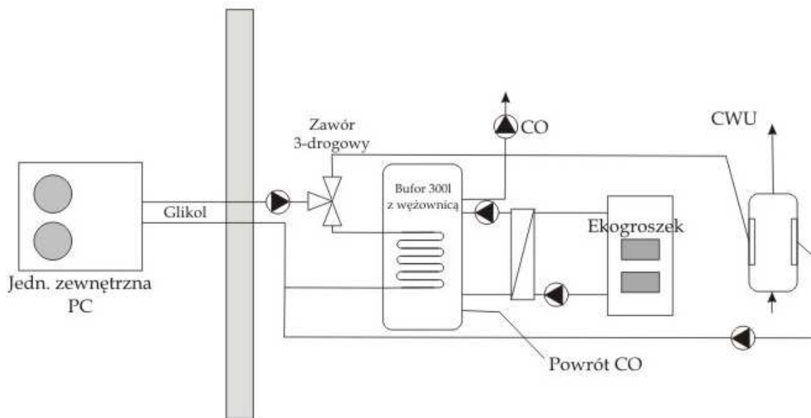
Schemat poglądowy powietrznej pompy ciepła
