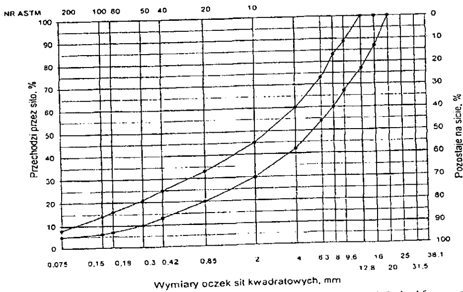
Rys. 13. Krzywe graniczne uziarnienia micszanki mineralnej BA od 0 do 16 mm do warstwy wyrównawczej nawierzchni drogi o obciążeniu ruchem od KR3 do KR6
