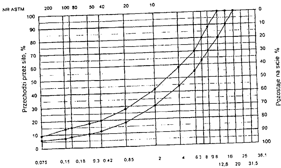
Rys. 6. Krzywe graniczne uziarnienia mieszanki mineralnej BA od 0 do 16 mm do warstwy ściaralnej nawierzchni drogi o obciążeniu ruchem od KR3 do KR6
