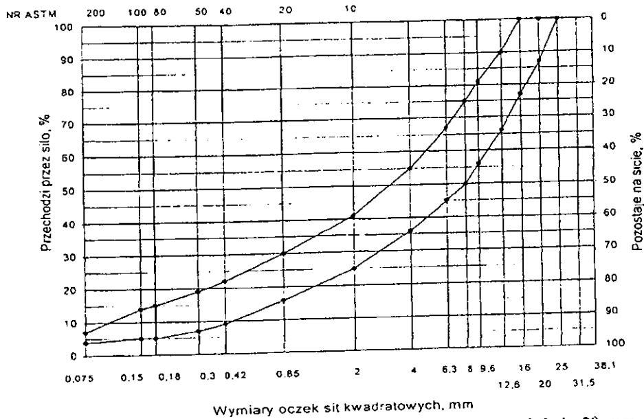
Rys. 12. Krzywe graniczne uziarnienia micszanki mineralnej BA od 0 do 20 mm do warstwy wiążącej, wyrównawczej i wzmacniającej nawierzchni drogi o obciążeniu ruchem od KR3 do KR6
