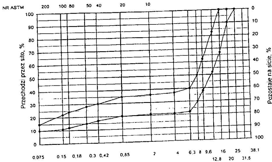
Rys. 5. Krzywe graniczne uziarnienia mieszanki mineralnej BA od 0 do 20 mm (mieszanka o nieciągłym uziarnieniu) do warstwy ściaralnej nawierzchni drogi o obciążeniu ruchem od KR3 do KR6
