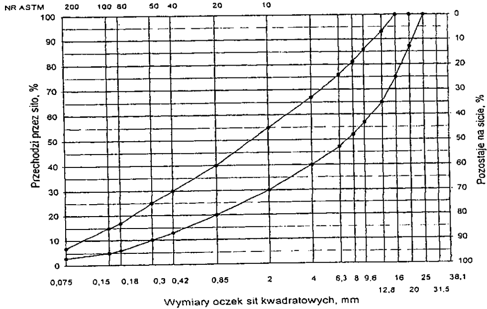
Rys. 8. Krzywe graniczne uziarnienia mieszanki mineralnej BA od 0 do 20 mm do warstwy wiążącej, wyrównawczej i wzmocniającej nawierzchni drogi o obciążeniu ruchem KRI lub KR2
