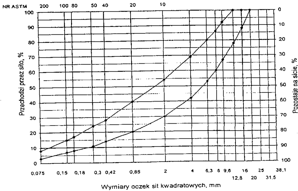
Rys. 9. Krzywe graniczne uziarnienia mieszanki mineralnej BA od 0 do 16 mm do warstwy wiążącej, wyrównawczej i wzmocniającej nawierzchni drogi o obciążeniu ruchem KRI lub KR2
